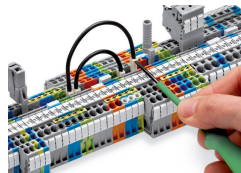
Leitungsbrücker bis zum Anschlag hinunterdrücken. Für Umverdrahtungen Briicker mittels Betätigungswerkzeug heraushebeln.
