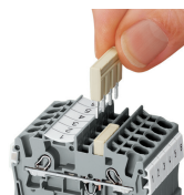
Kammbriicker einsetzen und bis zum Anschlag hinunterdrücken.
