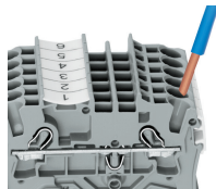
Leiter anschließen – direkt stecken. Eindrähtige Leiter lassen sich bis zu einem Querschnitt über und mindestens zwei Querschnittstufen unter dem Nennquerschnitt direkt stecken ohne Werkzeug.
