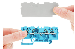
Trennwand Ex e/Ex i Die erste Klemme nach einer Trennwand Ex e/Ex i ist mit einer Abschlussplatte zu versehen!
