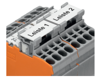
Der Beschriftungsadapter für Beschriftungsstreifen (2002-161) ist in die Brückeroöffnungen einsetzbar.
