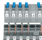
Die Prüfsteckermodule werden direkt in die Brückerschlitze der Stromschiene gesteckt (hier Serie 284).
