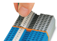
Beschriftung mit WMB-Multibeschriftungssystem
