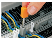
Prüfen mit Prüfstecker Hier über den Prüfadapter (209-170)
