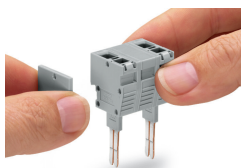
Zusammenrasten von Prüfstecker- und Blindmodulen zu mehrpoligen Prüfsteckerleisten (max. 10-polig) für Klemmenbreite 10 mm
