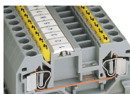
In die Betätigungsöffnungen eingesetzte Warnabdeckungen
