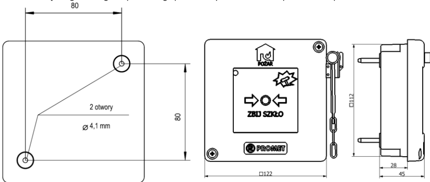
Rys. 1. Rozstaw otworów do mocowania oraz wymiary gabarytowe ręcznego ostrzegacza pożarowego ROP-A
