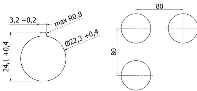
Rys2. Otwór montażowy oraz minimalne odległości pomiędzy montowanymi napędami.
