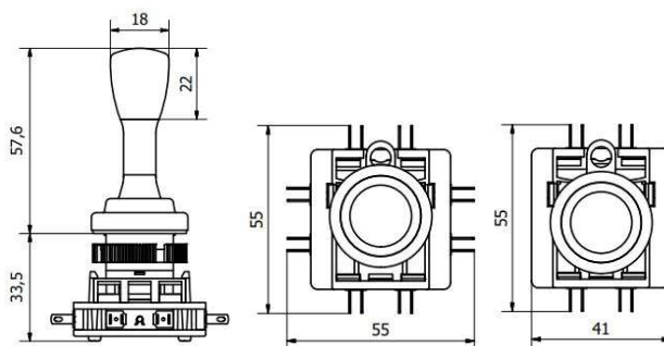
Rys3. Rysunek wymiarowy
