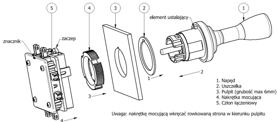
Rys1 . Montaż do pulpitu
