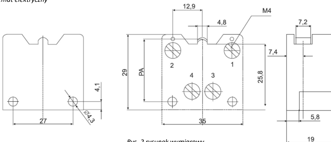
Rys. 2 rysunek wymiarowy
