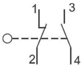
Rys. 1 schemat elektryczny
