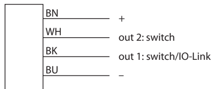
Fig. 13: CMMT-QR20-IOLX3 wiring diagram
