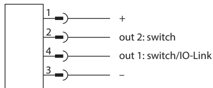
Fig. 12: CMMT-QR20-IOLX3-H1141 and CMMT-QR20-IOLX3-0.3-RS4 wiring diagram
