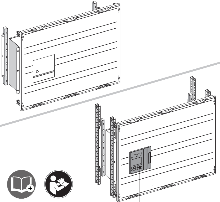
ATS TruONE-500A-800A-3/4p
