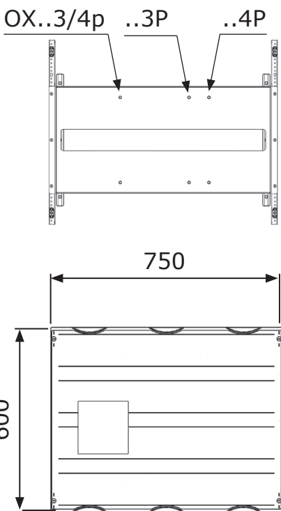
ATS TruONE-500A-800A-3/4p
