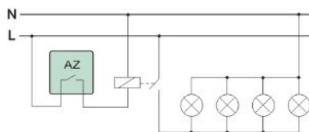
Układ sterowania stycznikiem załączającym odbiorniki o łącznym poborze prądu przewyższającym dopuszczalne obciążenie styku automatu zwierzcowego
