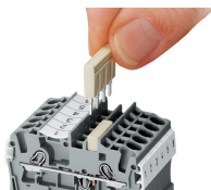
Kammbrücken einsetzen und bis zum Anschlag hinunterdrücken.
