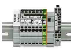
Dieser speziell für die Herstellung einer Dreieckschaltung entwickelte Dreieckbrücken findet bei Motorklemmenbrettern mit Reihenklemmen TOPJOB® S seinen Einsatz.
