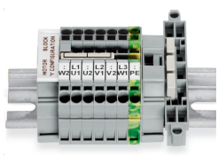
Dieser speziell für die Herstellung des „Sternpunktes“ entwickelte Sternbrücken findet bei Motorklemmenbrettern mit Reihenklemmen TOPJOB® S seinen Einsatz.
