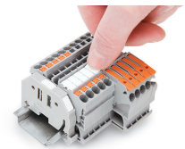
Einrasten eines WMB-Beschriftungsstreifens in die Beschriftungsaufnahme
