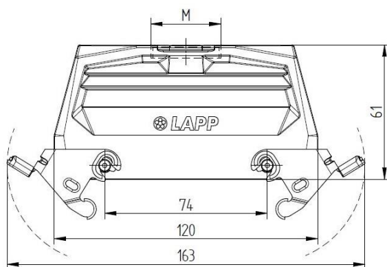
Kabeleingang gerade
