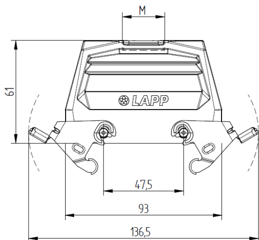
Kabeleingang gerade
