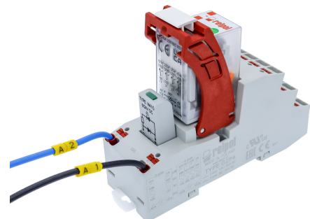
R4B-...-B in socket GZP4
