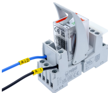
R4B-...-B in socket GZT4
