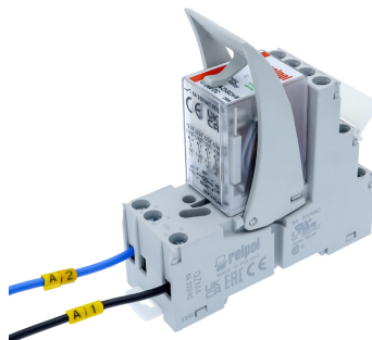
R4B-...-B in socket GZM4
