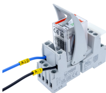
R4B-...-B w gnieździe GZT4
