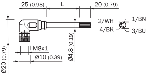
Rysunek wymiarowy (Wymiary w mm)
