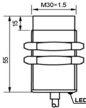
wyjście kablowe / cable output
