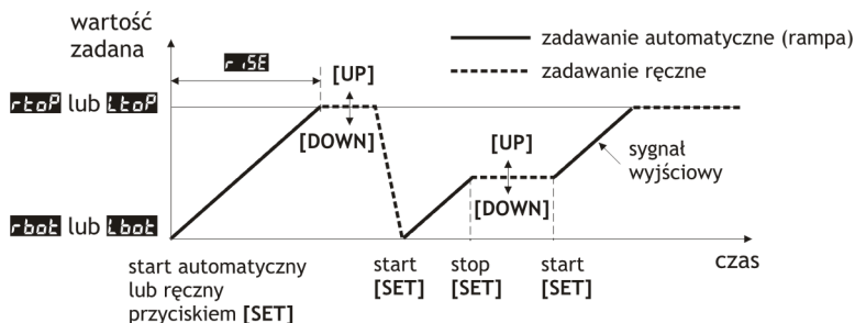
Rys. 11.1. Zasada działania wyjść w trybie miękkiego start (parametr rSE > 0, FRLL = OFF ).
