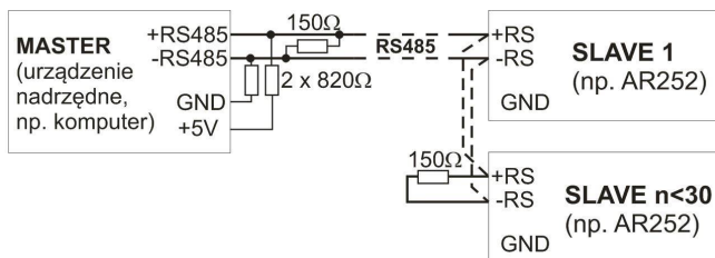
Rys.12. Schemat poglądowy sieci RS485
