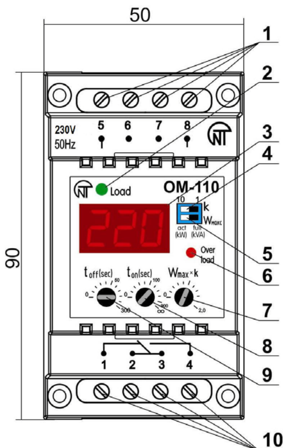
Rysunek 1 – Wygląd zewnętrzny OM-110
