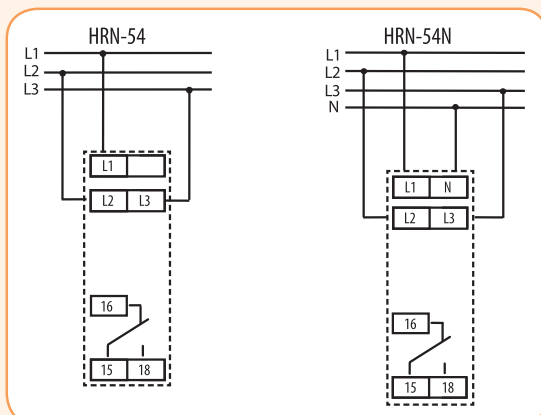
Układy połączeń
