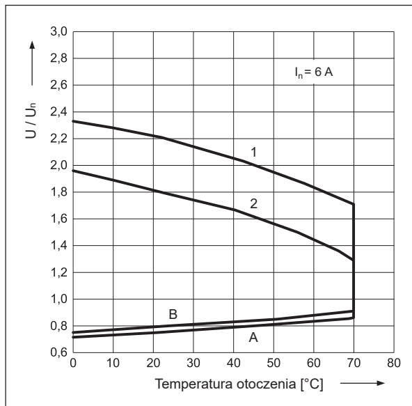
Dopuszczalny zakres napięcia pracy cewki - napięcie stałe Wykres 4
