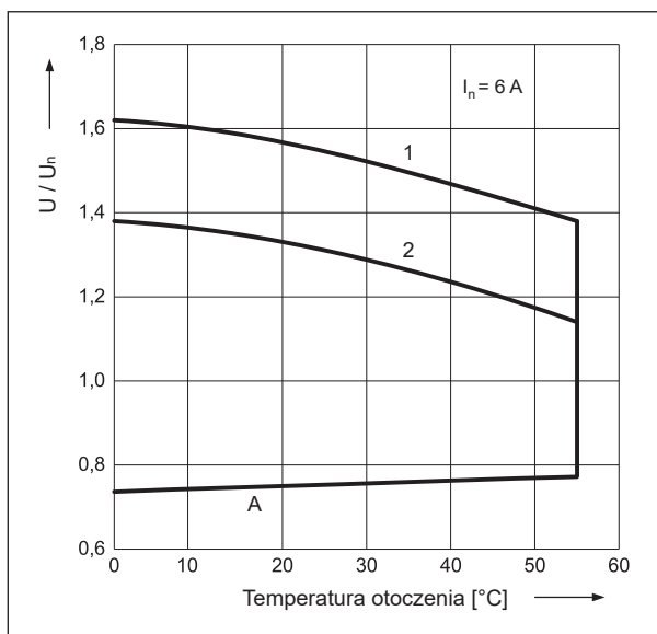
Dopuszczalny zakres napięcia pracy cewki - napięcie przemienne 50 Hz Wykres 5
