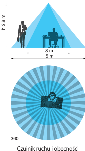
18.31...0031 - Montaż sufitowy wpuszczany lub powierzchniowy
