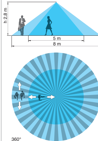
18.31...0031 - Montaż na wysokim suficie
