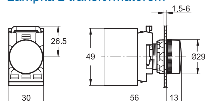
Lampka z transformatorem
