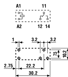
Rysunek otworów montażowych
