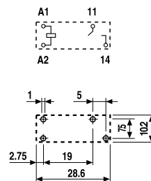
Rysunek otworów montażowych
