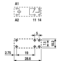
Rysunek otworów montażowych
