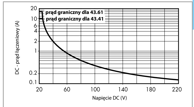
H 43 - Graniczna zdolność rozłączeniowa (dla DC1)
