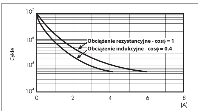
F 39 - Trwałość łączeniowa (dla AC) w funkcji prądu na zestykach
